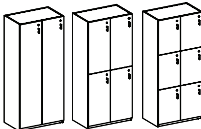
2-cluster
