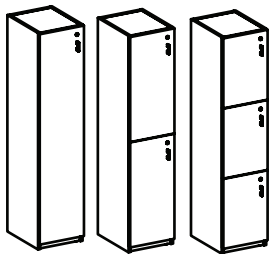
1-cluster
